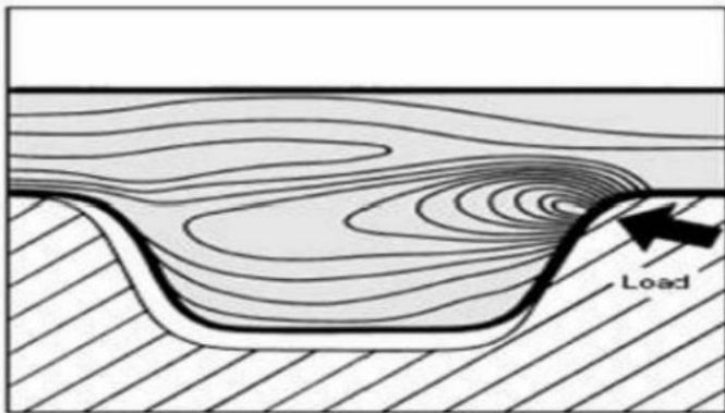
梯形皮带咬合状态与应力分布
