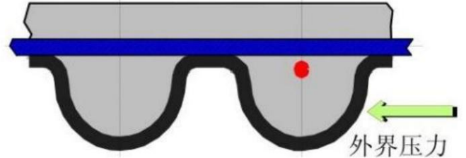
圆弧齿受力点
