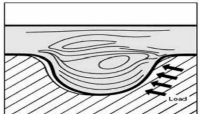
圆弧皮带咬合状态与应力分布
